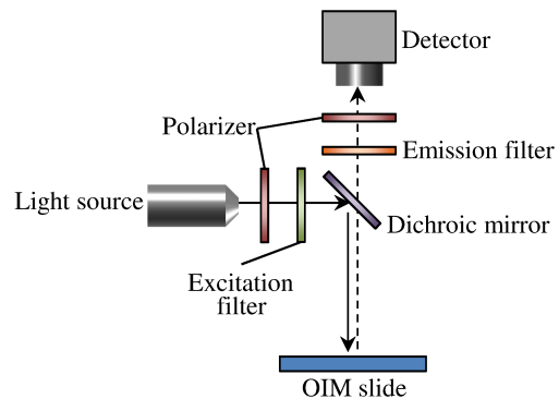
図6 タンパク質検出するための装置
